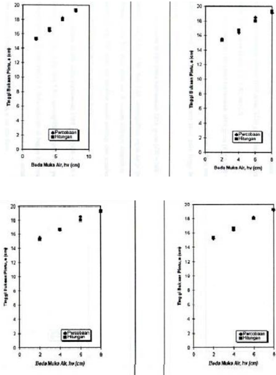
Gambar 6. Grafik Hubungan antara tinggi bukaan pintu dengan beda muka air berdasarkan sudut kemiringan (6a, 6b, 6c, 6d)
